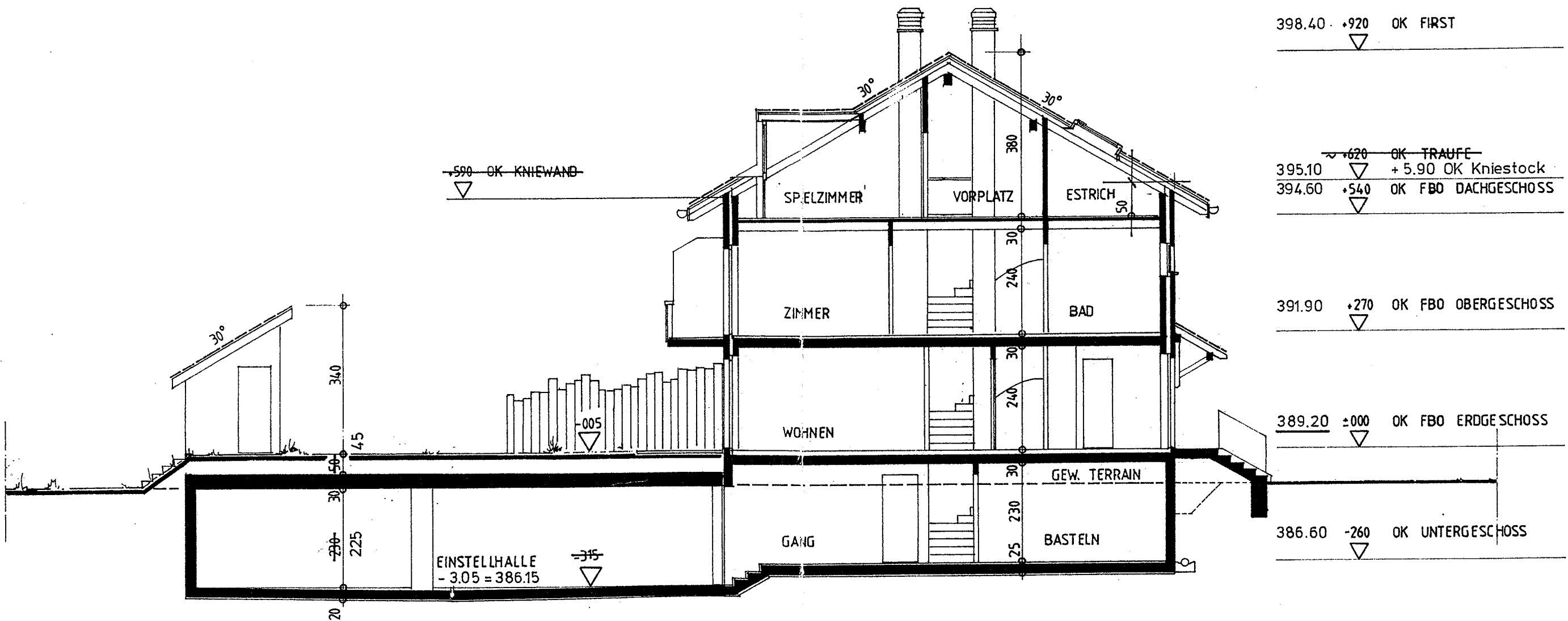
SCHNITT A-A
